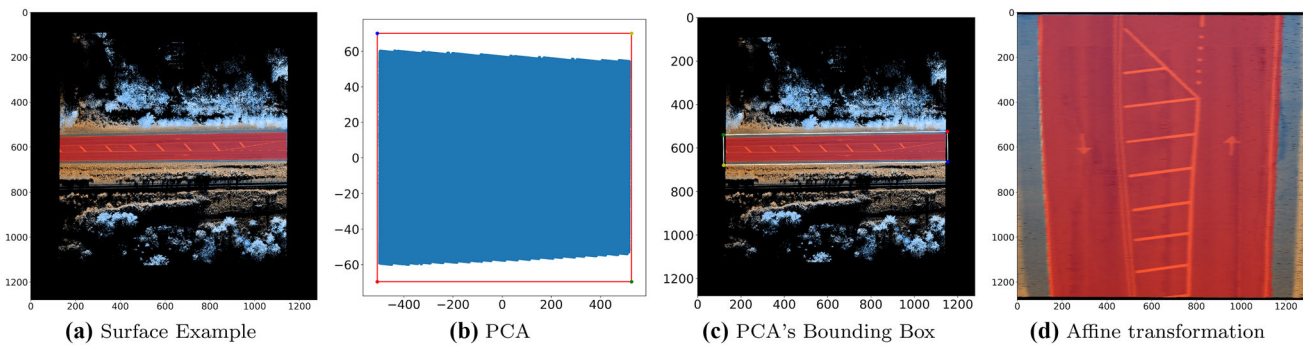
Fig. 5 PCA process
